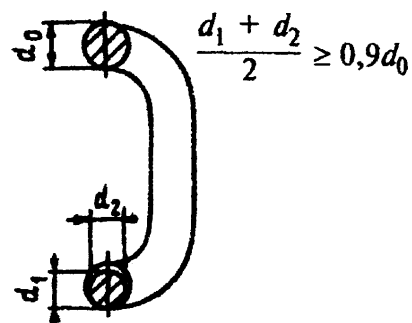
Рис. 2. Уменьшение диаметра сечения звена цепи: d_0 — первоначальный диаметр, мм; d_1, d_2 — фактические диаметры сечения, измеренные во взаимно перпендикулярных направлениях, мм
