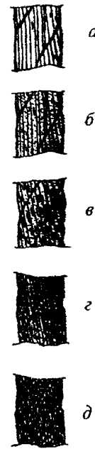
Рис. 6. Поверхностная коррозия проволок каната крестовой свивки: a — начальное окисление поверхности; б — общее окисление поверхности; в — заметное окисление; z — сильное окисление; д — интенсивная коррозия
